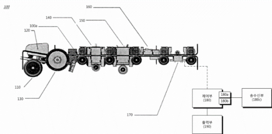
<하이브리드 위폐 감별 장치>
